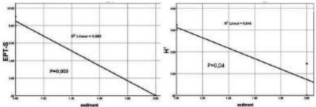
Grafikon 4. Regresijska analiza bioloških parametara (EPT-S i H') i tipa sedimenta Graph 4. Regression analysis of biological parameters (EPT-S and H') and sediment type
